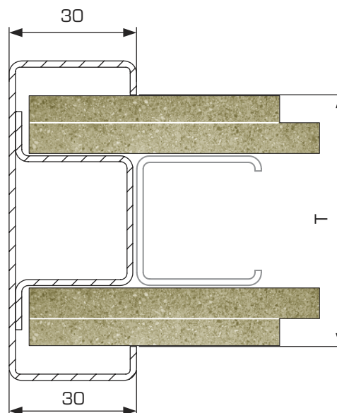
Řez obrubňového profilu pro SDK příčku
