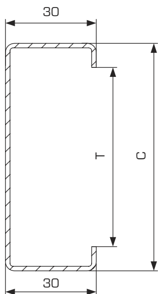
Řez obrubňového profilu pro zděnou příčku
