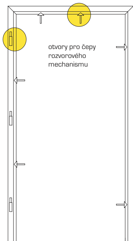
A) Zárubeň upravená pro bezpečnostní dveře
