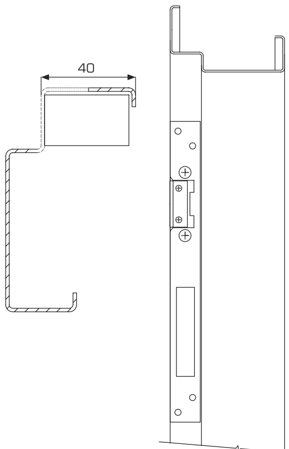
B) Zárubeň upravená pro instalaci elektromagnetického otevírače
